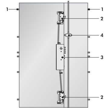
Bi-Elettro/Detector D.B.
