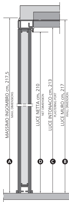
FRONTE E SEZIONE VERTICALE Front and vertical section
