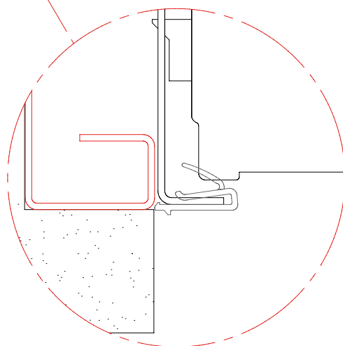
GUARNIZIONE STANDARD - STANDARD GASKET (ALIAS 1)
