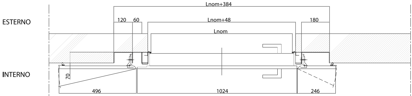
Sezione quotata Larghezza dim. nom. 900 mm
