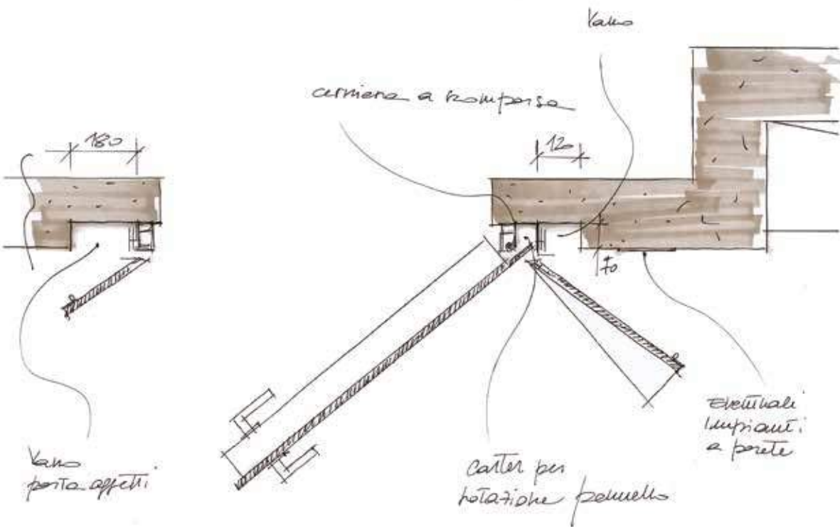
UN ESEMPIO DI COME RISULTA SEMPLICE INSERIRE IL SISTEMA WING ALI IN UN VANO PORTA, DI NUOVA COSTRUZIONE OPPURE IN UNA RISTRUTTURAZIONE.
